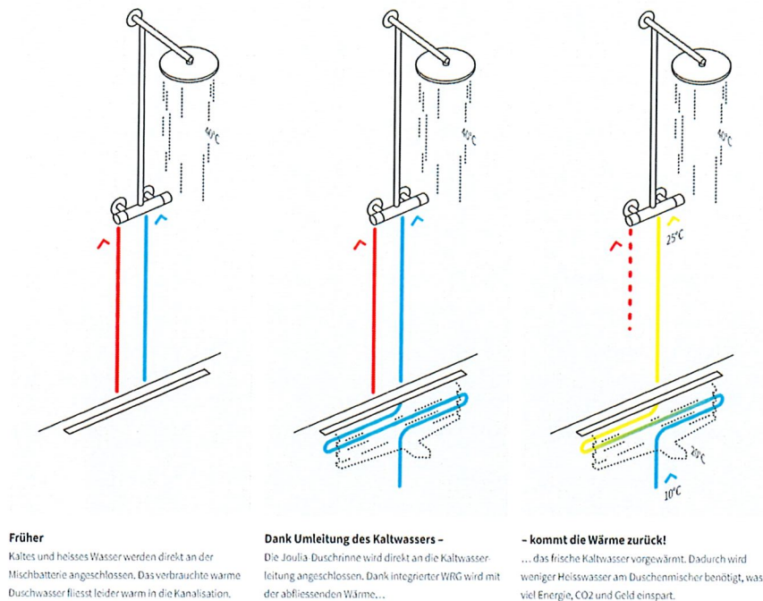
Abbildung 3: Prinzip der Joulia-Duschrinne (Quelle: www.joulia.com )
